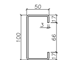
DETALHE PERFIL U TERÇAS Esc. 1:5
