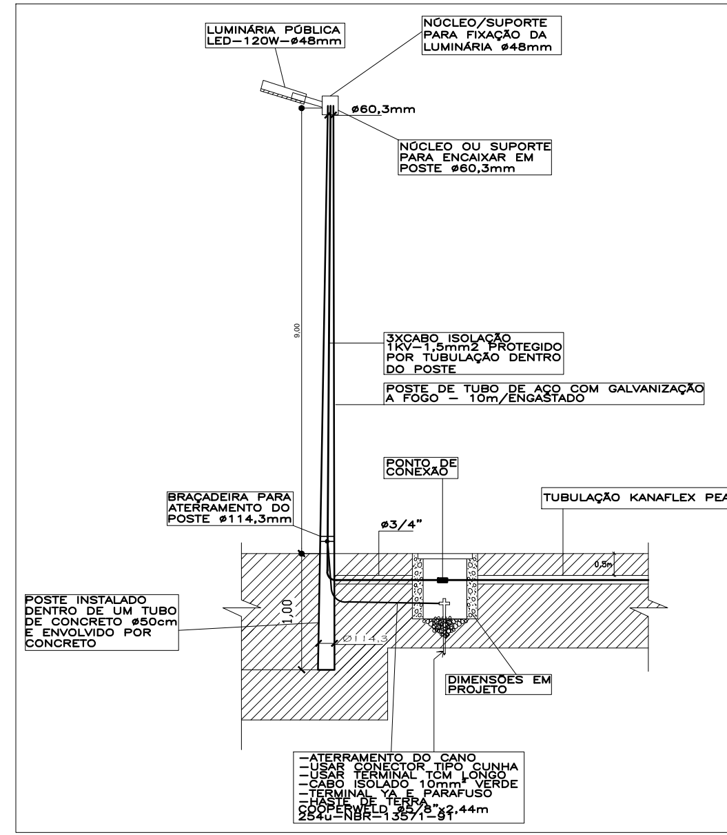
DETALHE DA ILUMINAÇÃO 1(UMA) PÉTALA
