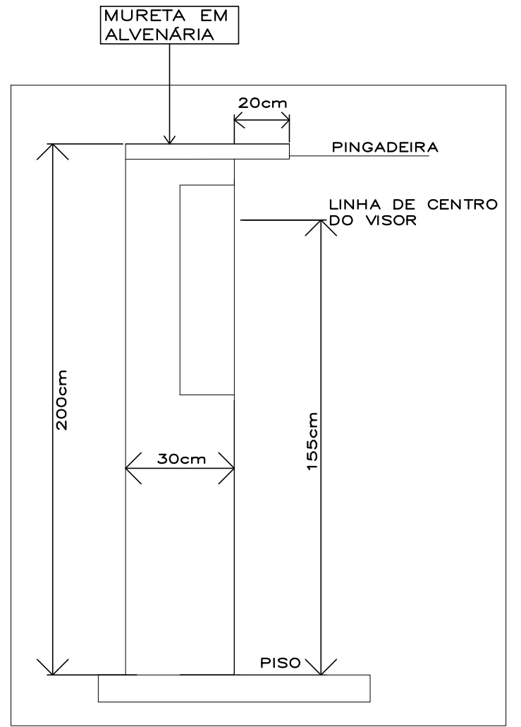
DETALHE DA INSTALAÇÃO DA CAIXA EXTERNA DE MEDIÇÃO EMBUTIDA EM MURETA DE ALVENARIA
