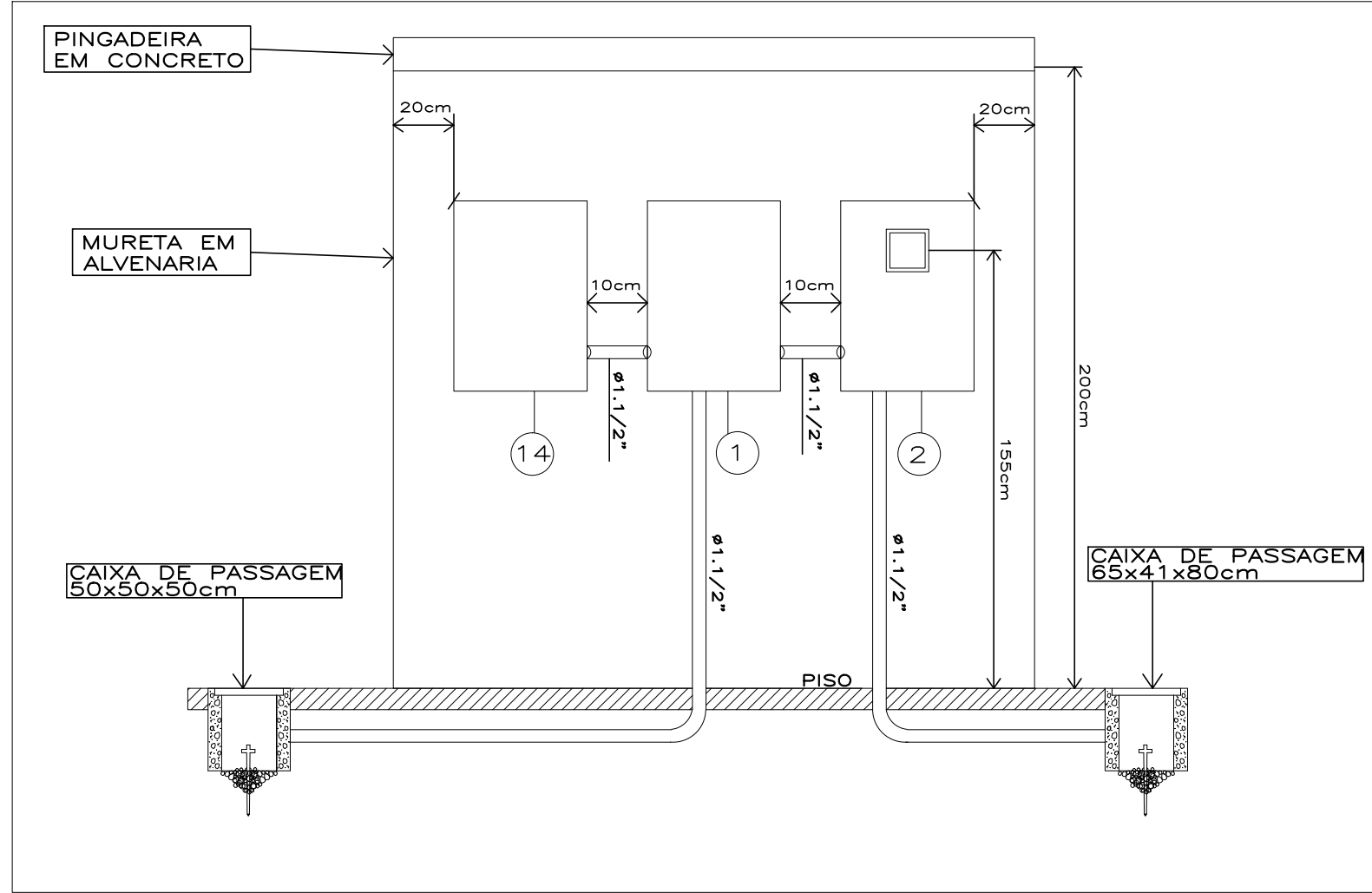
DETALHE DA MURETA EM ALVENARIA CAIXA DO MEDIDOR CAIXA DE PROTEÇÃO E DISTRIBUIÇÃO CAIXA COM AS TOMADAS
