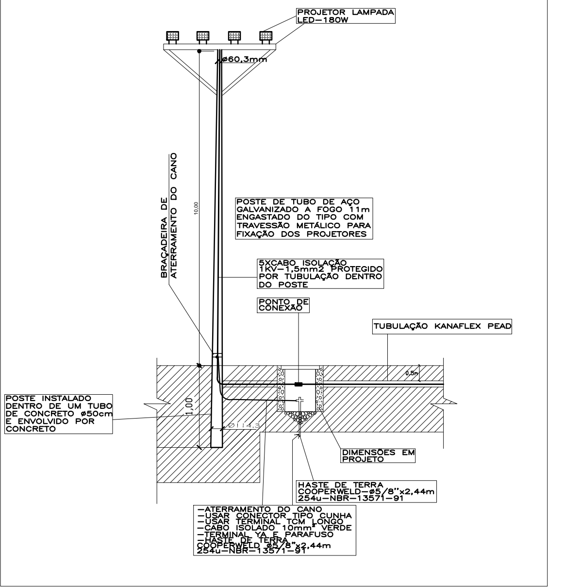
DETALHE DA ILUMINAÇÃO PROJETORES DO CAMPO
