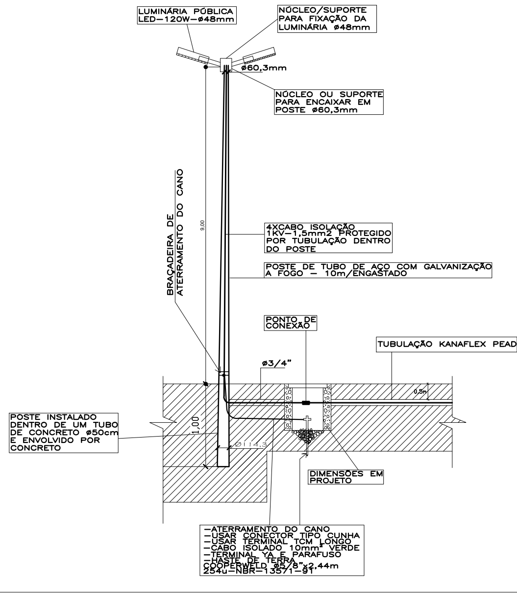
DETALHE DA ILUMINAÇÃO 2(DUAS) PÉTALAS
