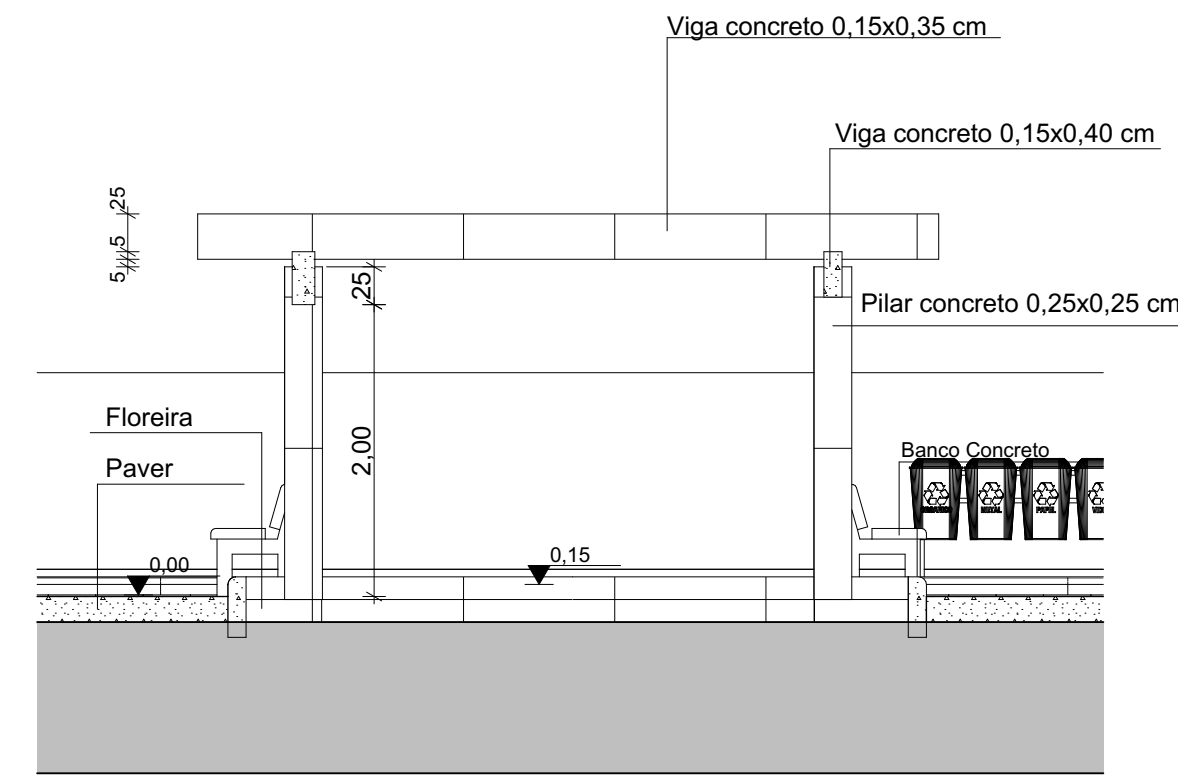
PÉRGOLAS -CORTE DD 1:50 (nivel específico)
